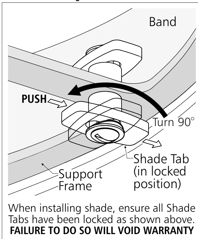
Fig. 9 - Shade Tab
